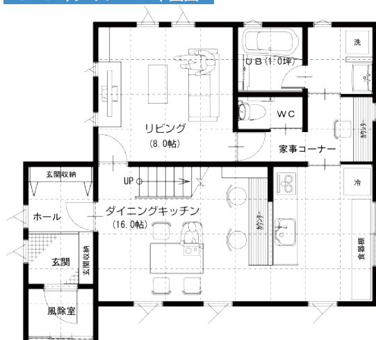
34.5 坪タイプ 1F 平面図
