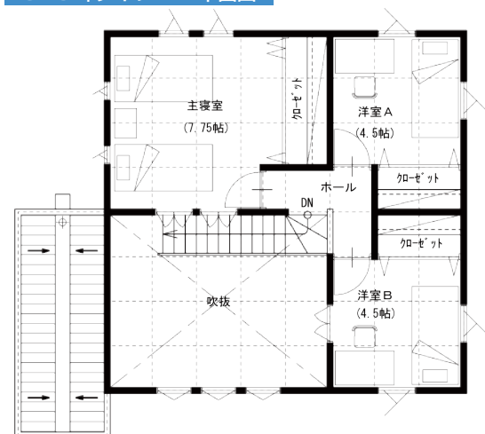
34.5 坪タイプ 2F 平面図
